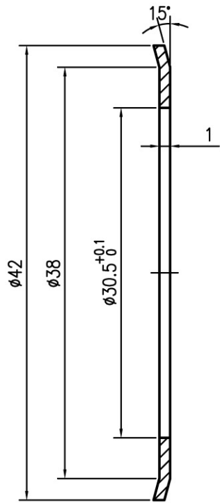
FLANGE 13#
